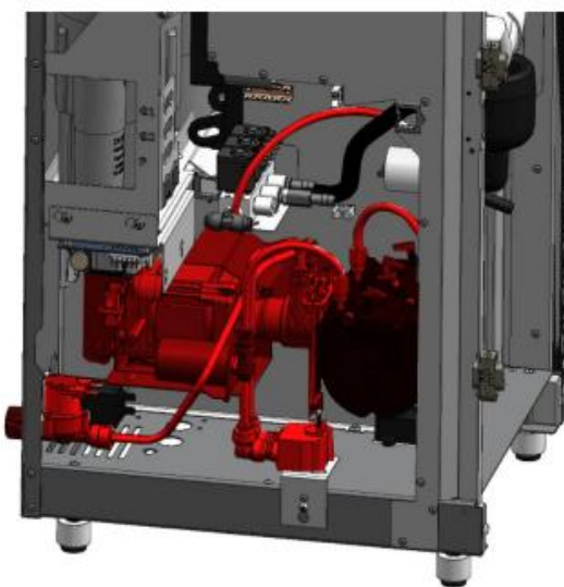
Nieuwe configuratie van het watercircuit
